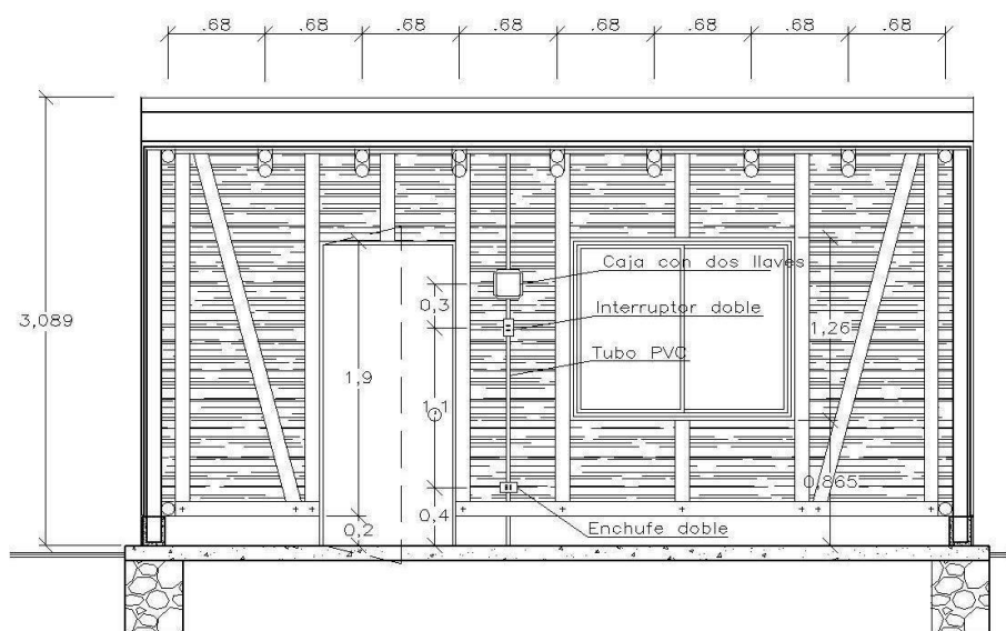
Corte 3-3
