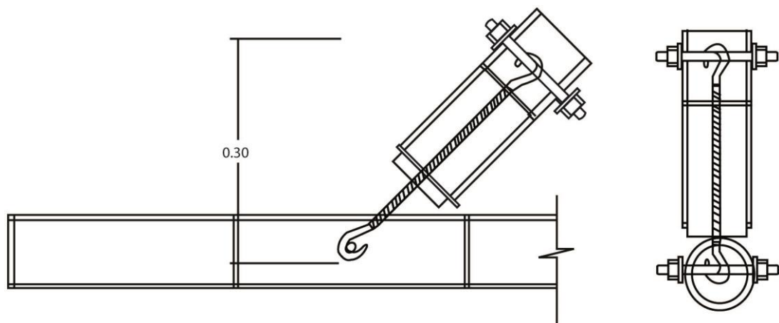
Corte
