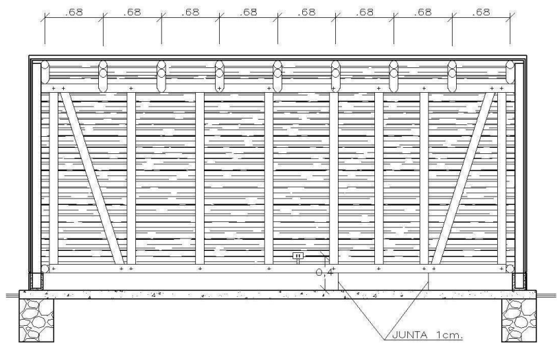
Corte 2-2
