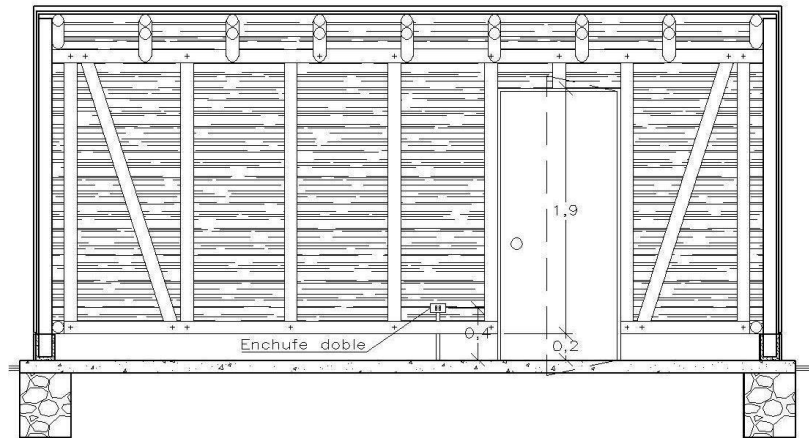
Corte 4-4
