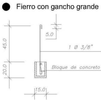
Detalle 2
