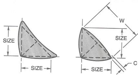
A) Perfiles de Soldadura de Filete Deseables
