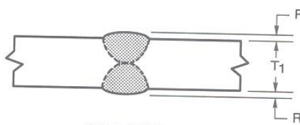
UNION A TOPE – PLANCHAS DE IGUAL ESPESOR
