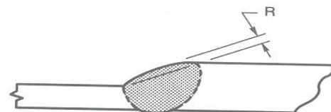
UNION A TOPE (TRANSICIÓN) PLANCHAS DE ESPESORES DESIGUALES
