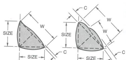
B) Perfiles de Soldadura de Filete Aceptables
