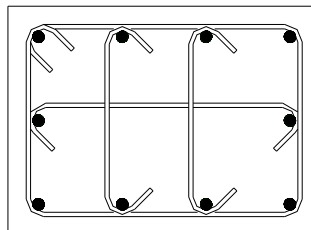
Un estribo y tres grapas suplementarias
