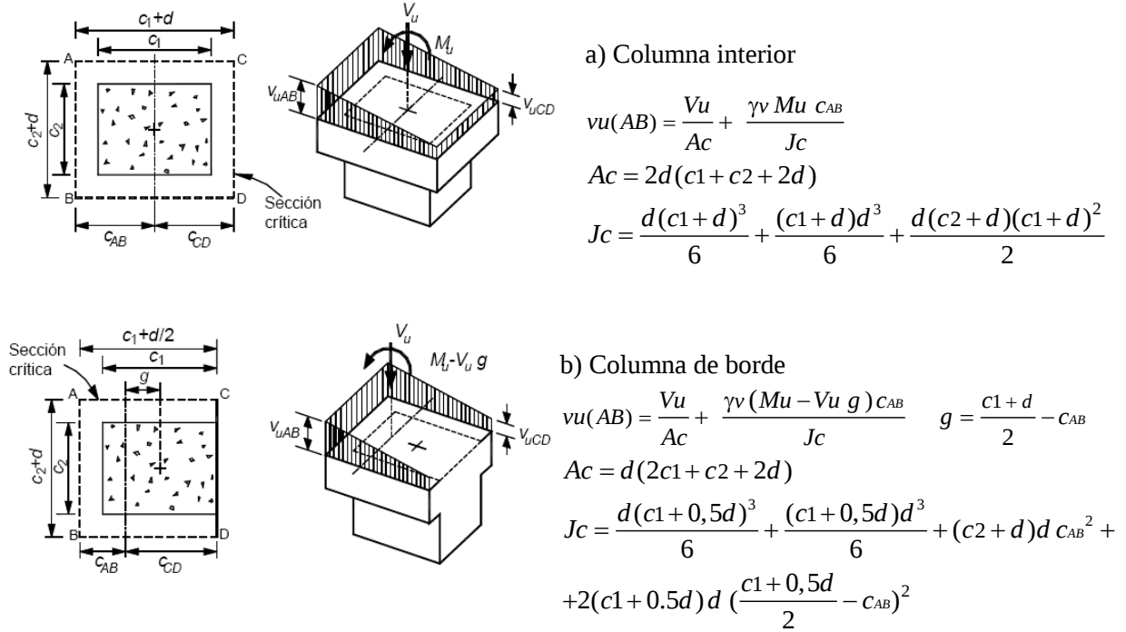
Fig. 11.12.6 Distribución de los esfuerzos cortantes en el perímetro de la sección crítica en conexiones losa a columna
