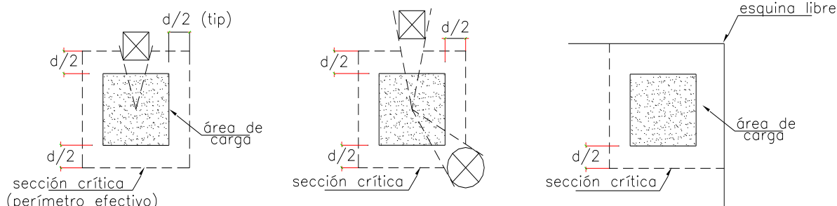
Fig. 11.12.5.1 Aberturas y bordes libres en losas (las líneas discontinuas muestran el perímetro efectivo).
