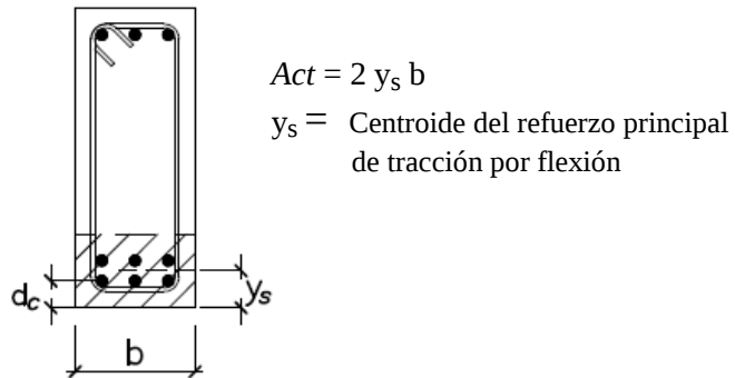
Fig. 9.9.3 Area efectiva de concreto en tracción.
