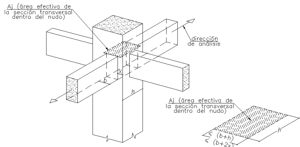
Fig. 21.7.4.1 Área efectiva en el nudo
