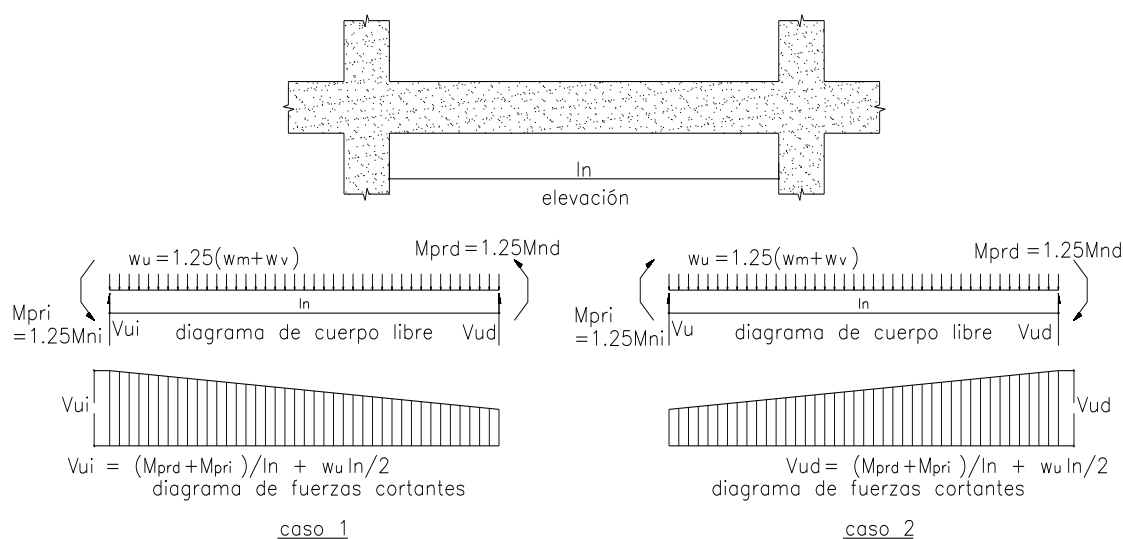
Fig. 21.5.4.1 Fuerza cortante de diseño en vigas
