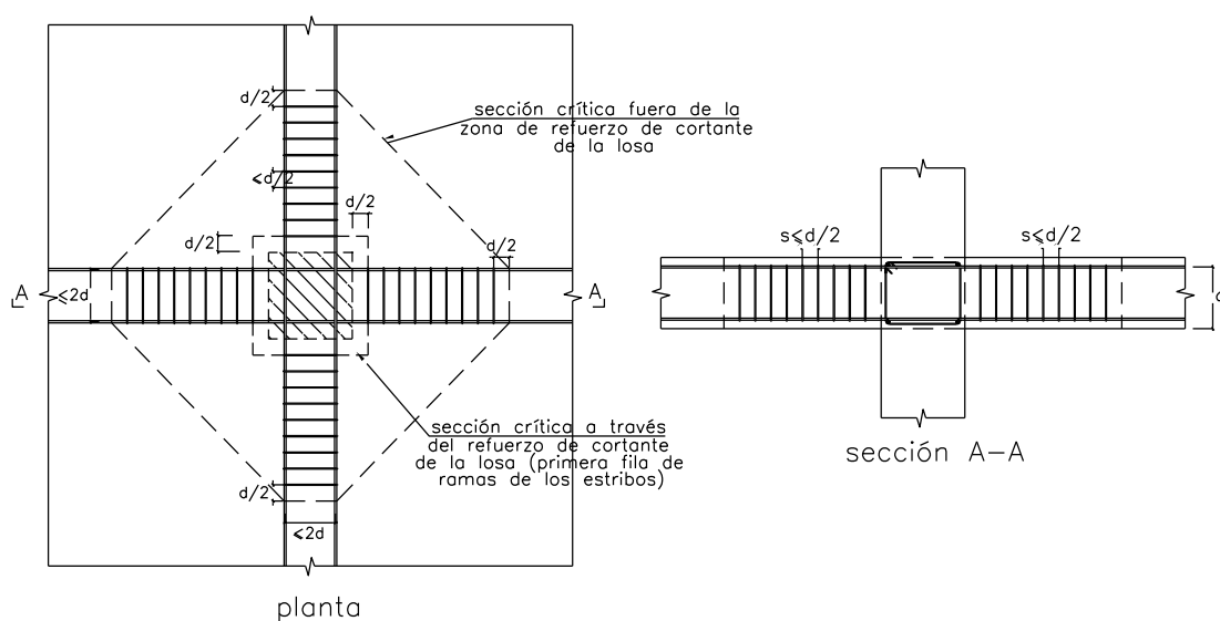
Fig. 11.12.3.a Disposición de los estribos por cortante en columnas interiores.
