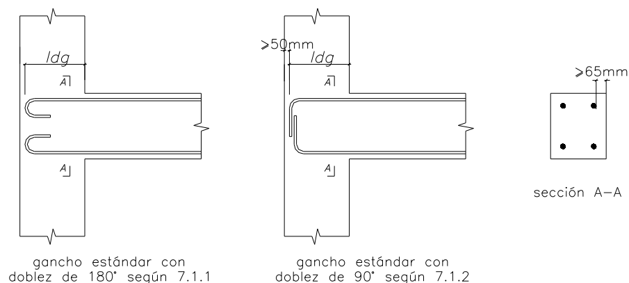
Fig. 12.5.3.a Casos en los que se puede multiplicar \ell_{dg} por 0,7
