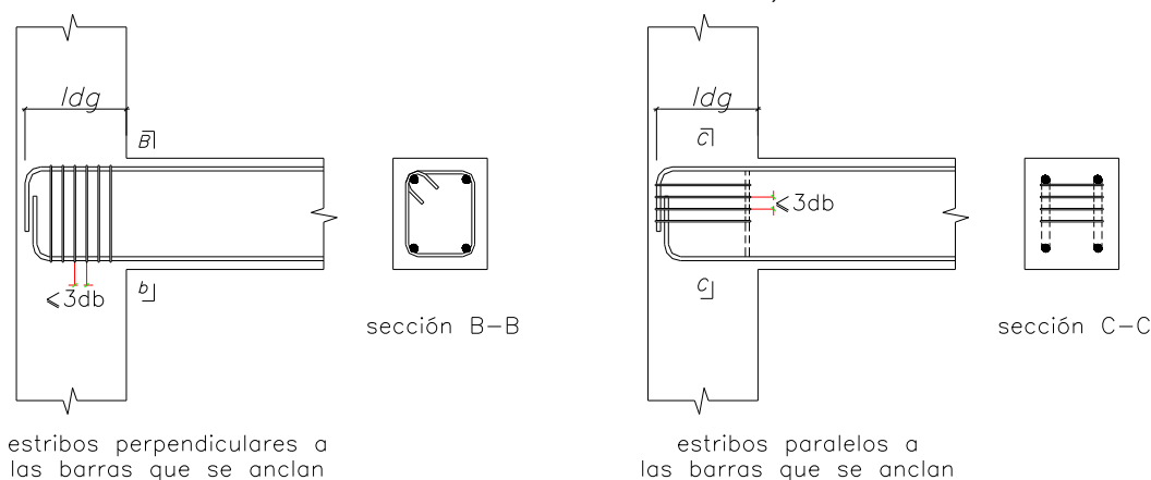
Fig. 12.5.3.b Casos con gancho estándar a 90° en los que se puede multiplicar \ell_{dg} por 0,8
