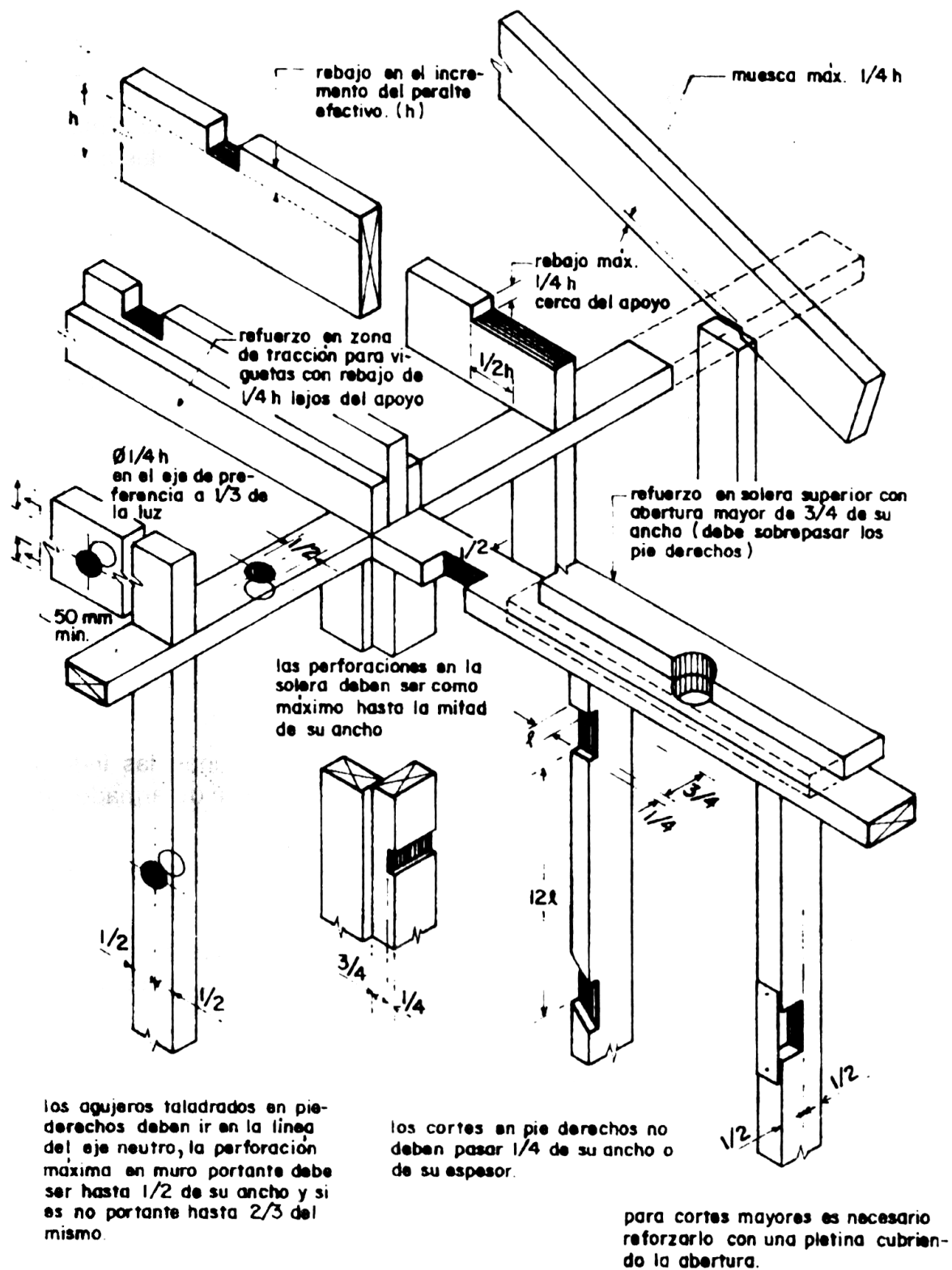
Fig. 12.2.2 Perforaciones y rebajos en elementos de madera.
