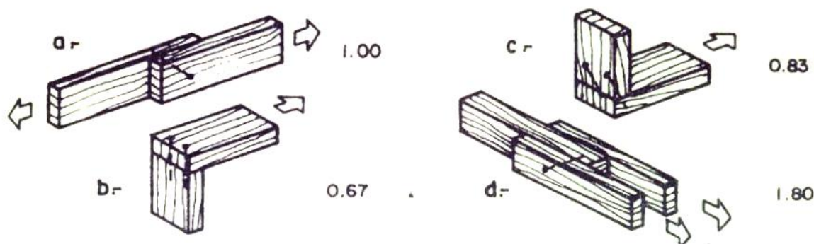
Fig. 10.2.3.1. Factores modificatorios de las cargas admisibles para uniones clavadas sometidas a cizallamiento simple.
