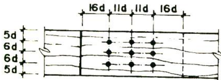
Fig. 10.2.5.3a Elementos cargados paralelamente al grano.
