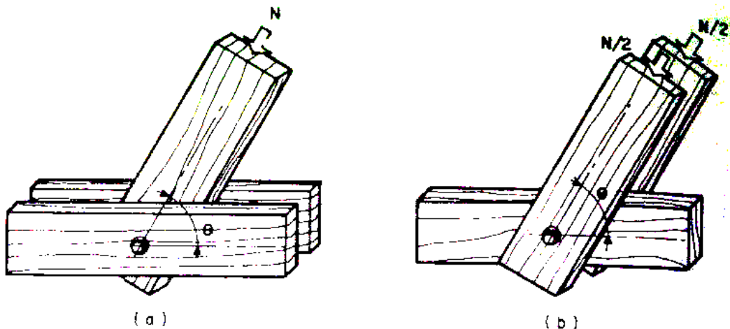
Fig. 10.3.2.3 Unión empernada, cargas inclinadas con relación al grano
