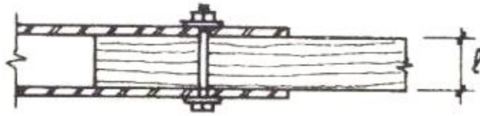
Fig. 10.3.2.4 Unión emperrada con pletinas metálicas
