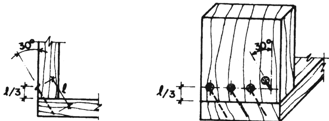
Fig. 10.2.4.1c Ubicación de clavos lanceros.
