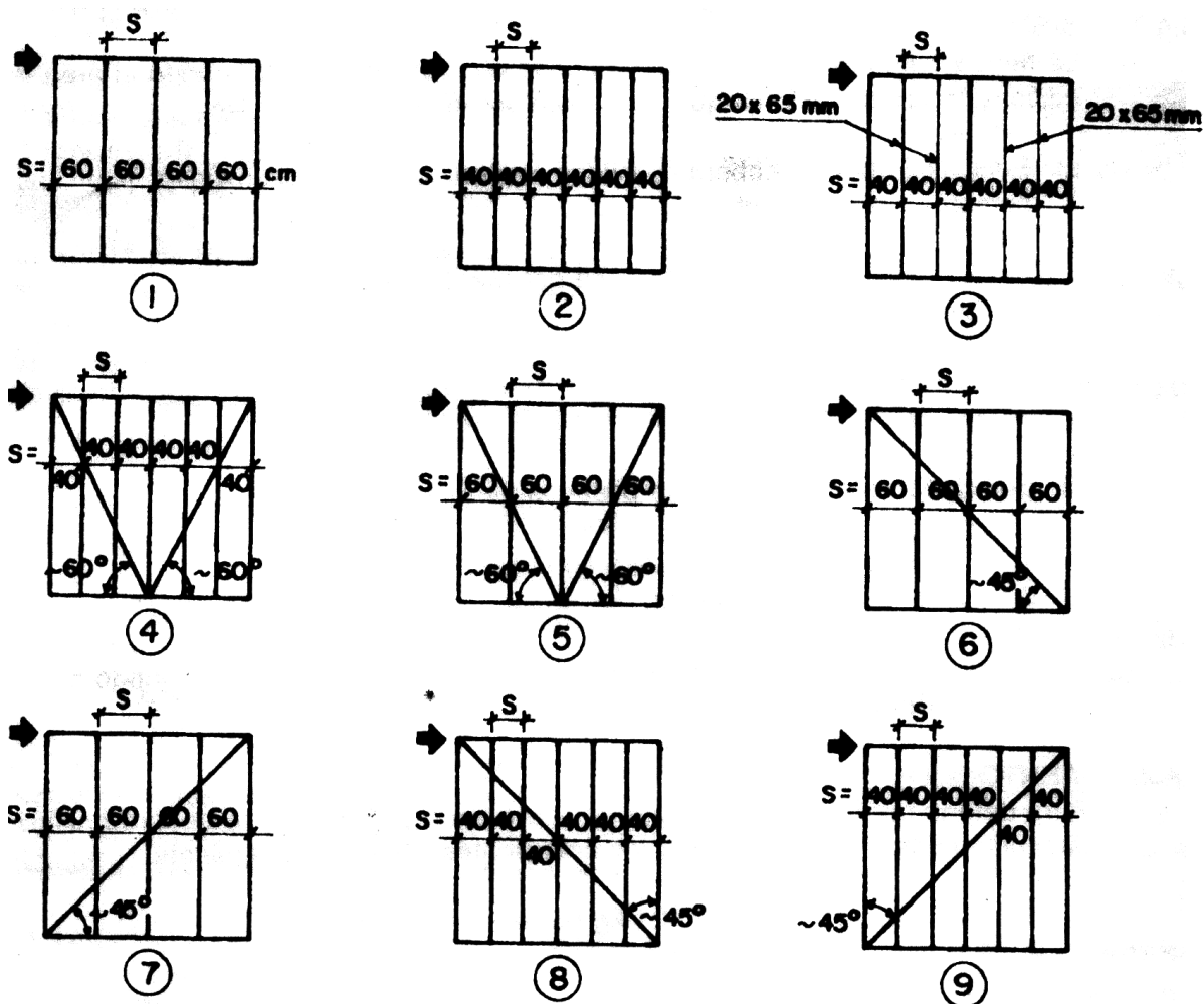
Fig. 8.6.1. Tipos de entramados.
