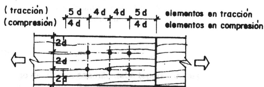
Fig. 10.3.3.3a Espaciamientos mínimos entre pernos, cargas paralelas al grano.
