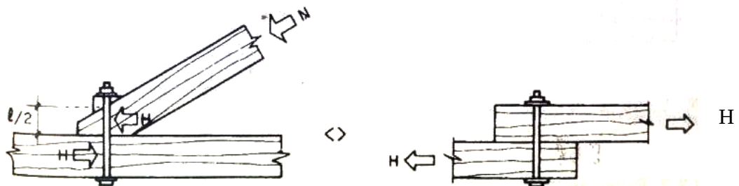
Fig. 10.3.2.7 Unión emperrada sometida a cizallamiento y fuerza axial
