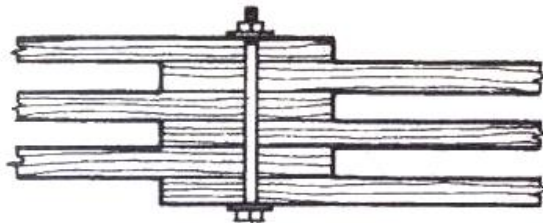
Fig. 10.3.2.6 Unión emperrada sometida a cizallamiento múltiple
