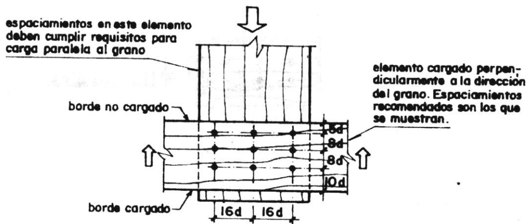
Fig. 10.2.5.2b Elementos cargados perpendicularmente al grano.
