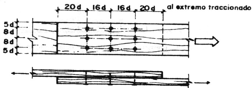
Fig. 10.2.5.2a. Elementos cargados paralelamente al grano.
