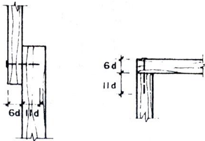
Fig. 10.2.4.1a Espesores mínimos y penetración de clavos sometidos a cizallamiento simple.
