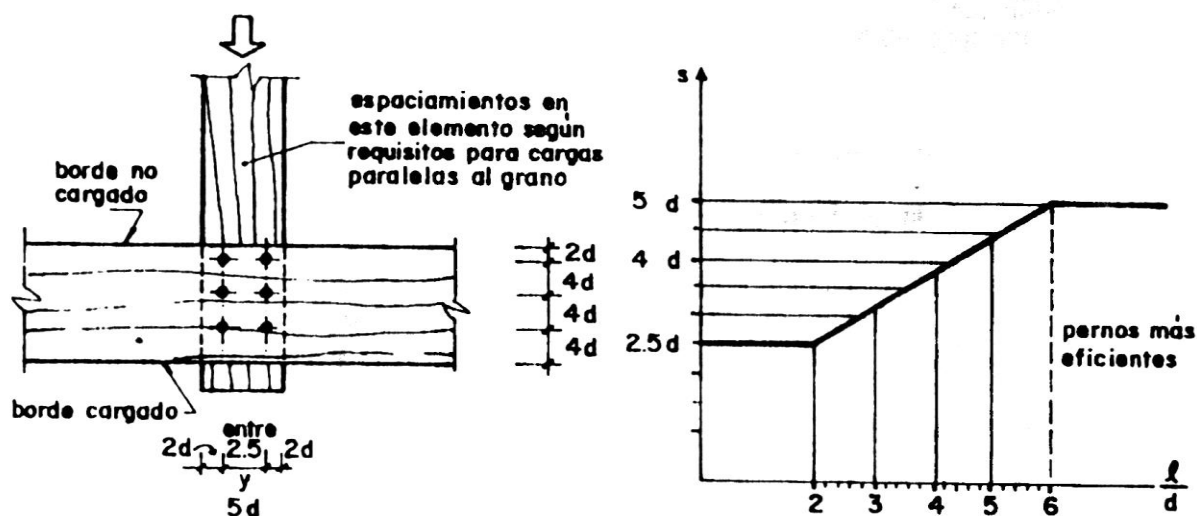
Fig. 10.3.3.3b Espaciamiento mínimo entre pernos, cargas perpendiculares al grano.
