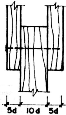
Fig. 10.2.4.2 Espesores mínimos y penetración de clavos sometidos a doble cizallamiento.
