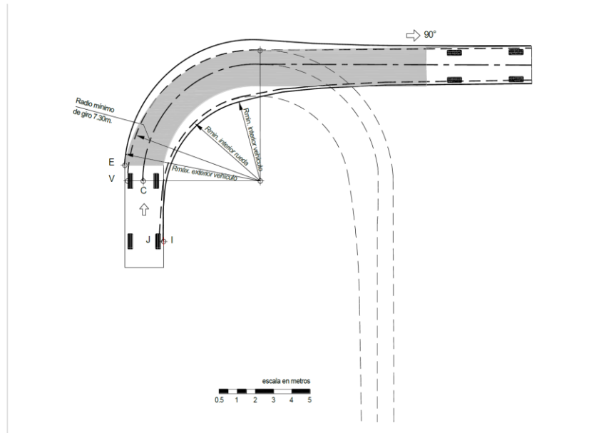
Esquema de giro de vehículo liviano
